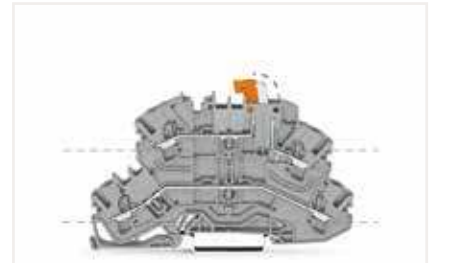
Bıçaklı ayrılmalı çift katlı ayırma klemensleri (2002-2671) Alt katta geçiş klemensleri, üst katta ayırma klemensleri olarak kullanılabilir.
