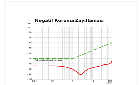
Blendaj bağlantı sistemi oldukça etkilidir çünkü sıkıştırma ünitesi kablunun blendajsız kısmına çok yaklaşılabılır.
